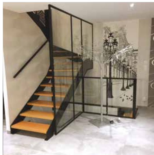
Ma-2 → Escalier 1/2 tournant avec marches en Hêtre sans contremarches, structure en limon «à la française», main-courante murale MC4 en acier thermolaqué, claustra vitré toute hauteur.
