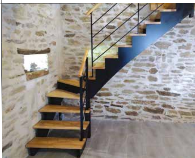
➤ Me-3 : Escalier 1/4 tournant en Frêne Olivier sans contremarches, sur crémaillères "à l'anglaise".
