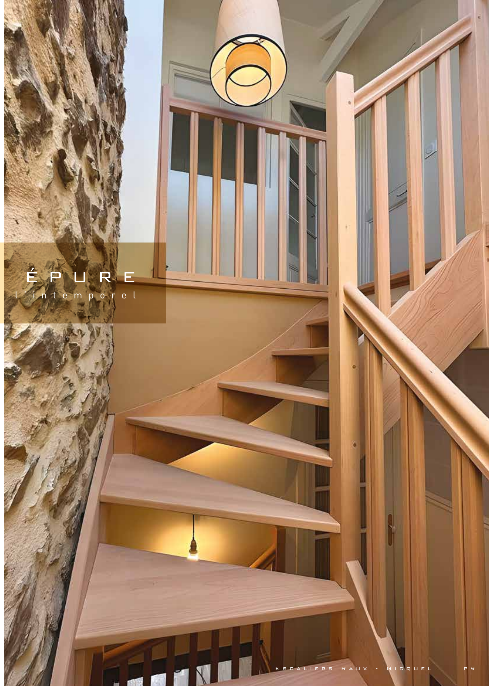
Ep-5 ➔ Escalier 2/4 tournant en Hêtre sans contremarches, poteaux T1, balustres G, main-courantes MC1, de conception traditionnelle avec crémaillère et plinthe murale massives.
